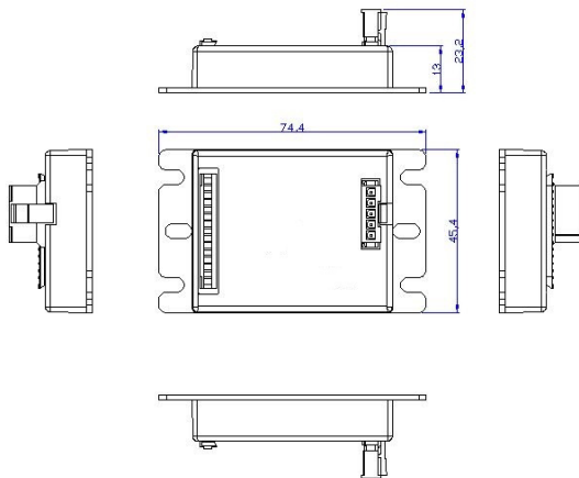
CANopen (Standard)
